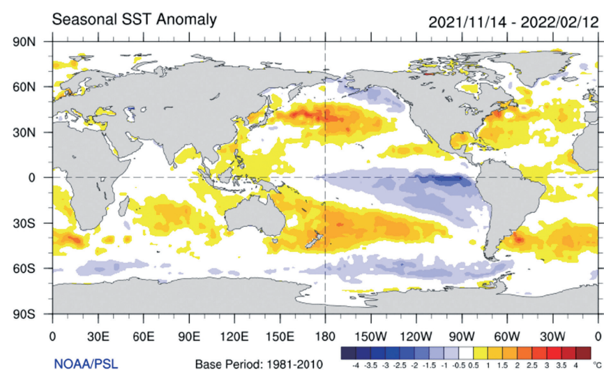
▲過去一季的海溫距平：反聖嬰現象成形。（賈新興提供）
