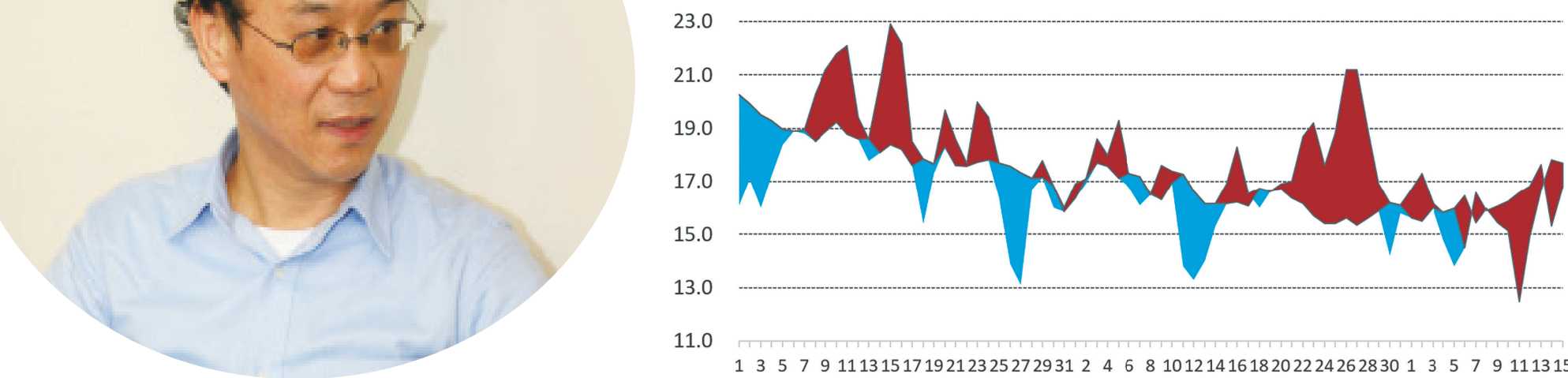
▲2021年12月1日至2022年2月15日台北氣象站日均溫和氣候值比較。（賈新興提供）
