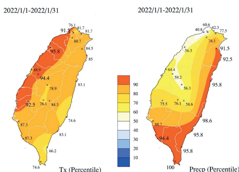
►2022年1月臺灣氣溫和降雨百分化分布圖。（賈新興提供）
