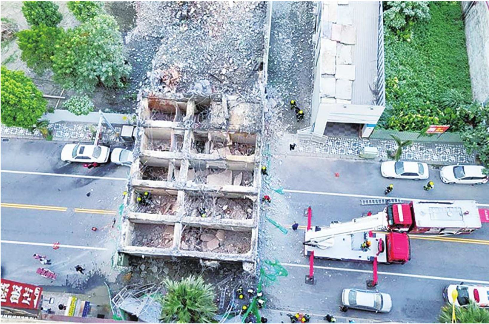
▲位在花蓮火車站前的「漫波假期飯店」大樓近日進行拆除作業，1日下午大樓驚傳倒塌，橫躺路面。(中央社)
