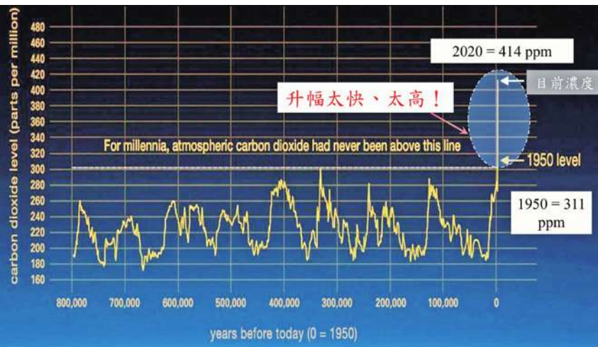
▲ 二氧化碳的濃度在大氣層的組成只有 0.041%，卻對地球氣候扮演舉足輕重的角色。（汪中和提供）
