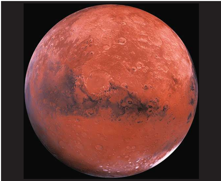
▲日前 NASA 的科學家首次偵測到火星的地震，再多一些記錄，科學家就能對火星的內部地質結構有更多了解。(pixabay)
