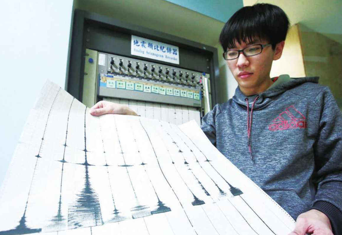
▲中央氣象局地震測報中心觀測，花蓮近海 6 日晚間 11 時 50 分發生芮氏規模 6.0 地震。圖為地震類比記錄器記錄下地震當時全台灣各地的地震波。(中央社)
