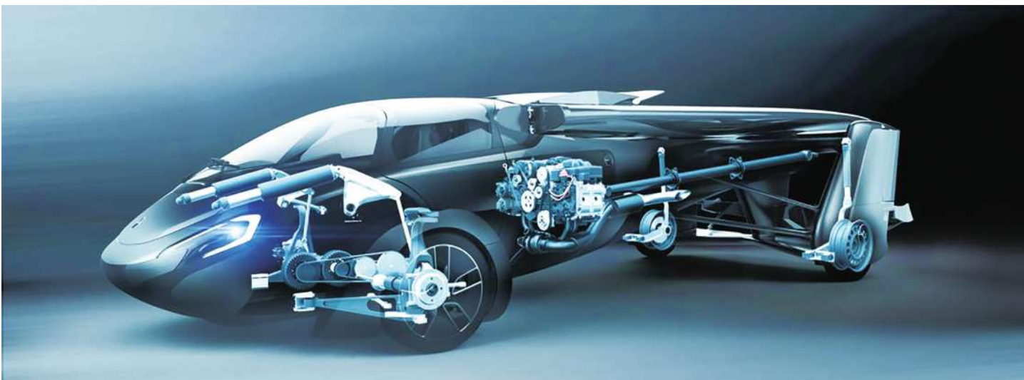
▲ AeroMobil 公司推出的飛天車造型。（圖：AeroMobil 官網）
