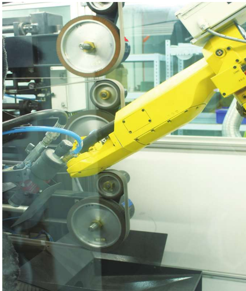
五軸復合加工機後,只要花10分鐘,就可以完成骨骼研磨。(photo by 譚有勝)
